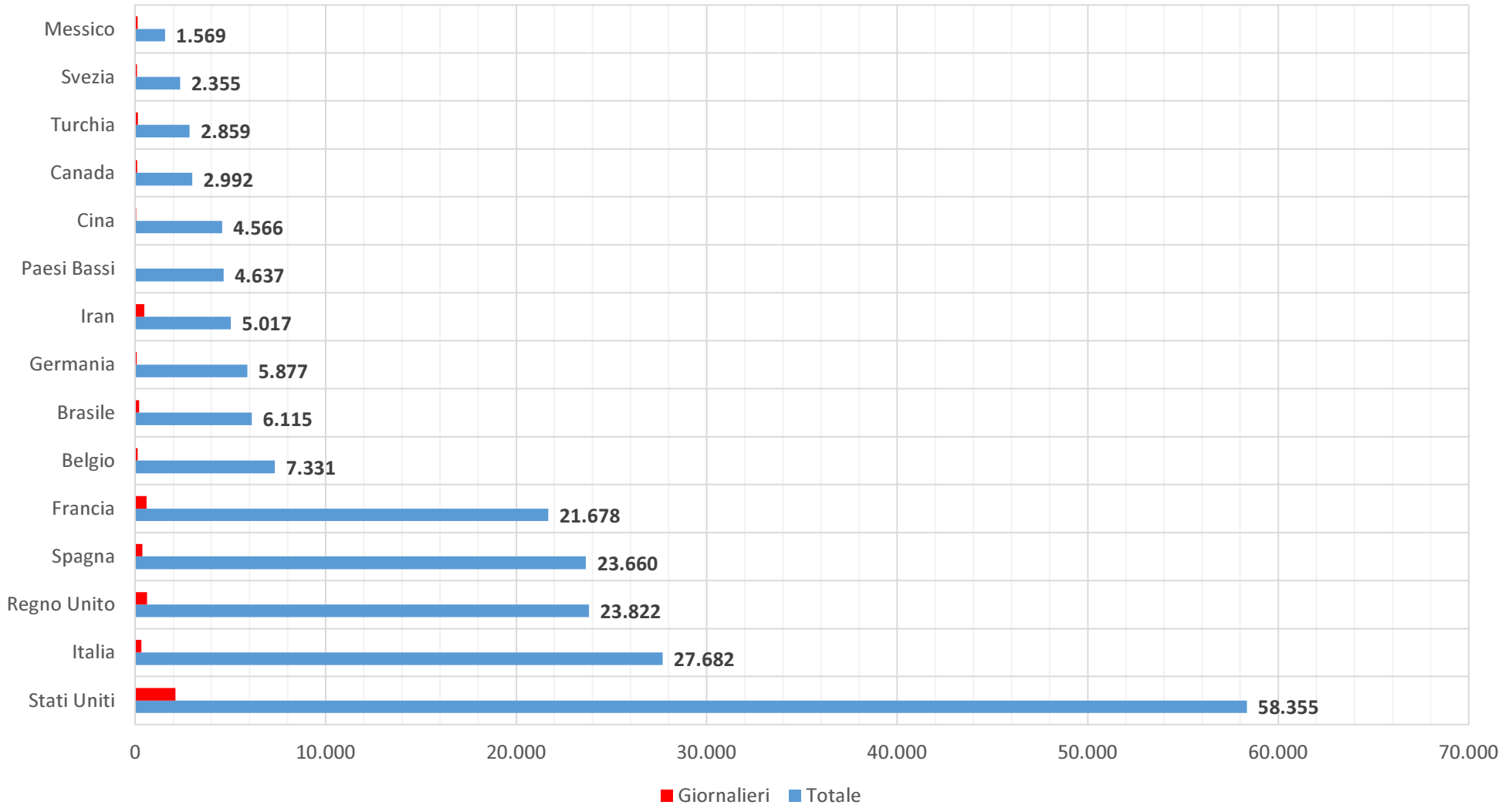
Fig. 12 - Numero totale e giornaliero di decessi nei paesi con più il più alto numero assoluto di decessi (dati del 4 maggio 2020)
