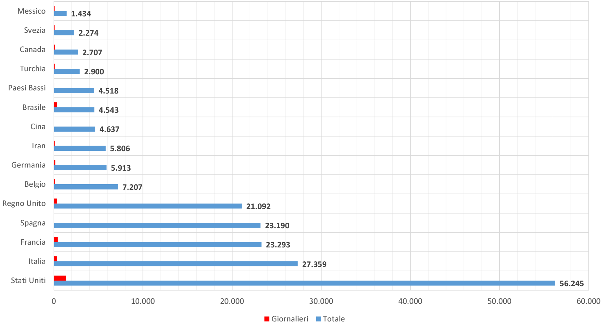
Fig. 12 - Numero totale e giornaliero di decessi nei paesi con più il più alto numero assoluto di decessi (dati del 28 aprile 2020)
