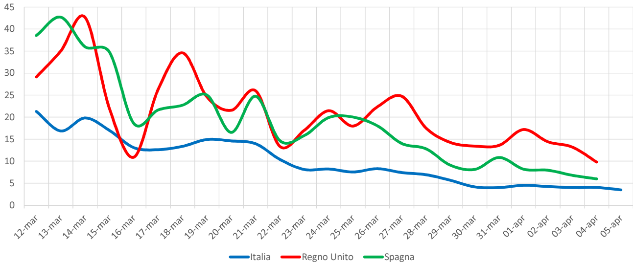
Fig. 10 - Confronto tra tasso di crescita giornaliero (%) del numero di contagiati confermati in 3 Paesi europei (dati del 5 aprile 2020)
