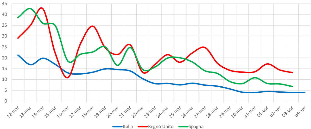
Fig. 10 - Confronto tra tasso di crescita giornaliero (%) del numero di contagiati confermati in 3 Paesi europei (dati del 4 aprile 2020)
