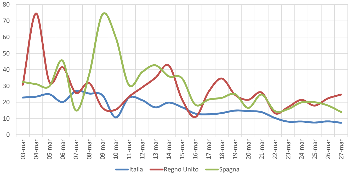
Fig. 10 - Confronto tra tasso di crescita giornaliero (%) del numero di contagiati confermati in 3 Paesi (dati del 28 marzo 2020)
