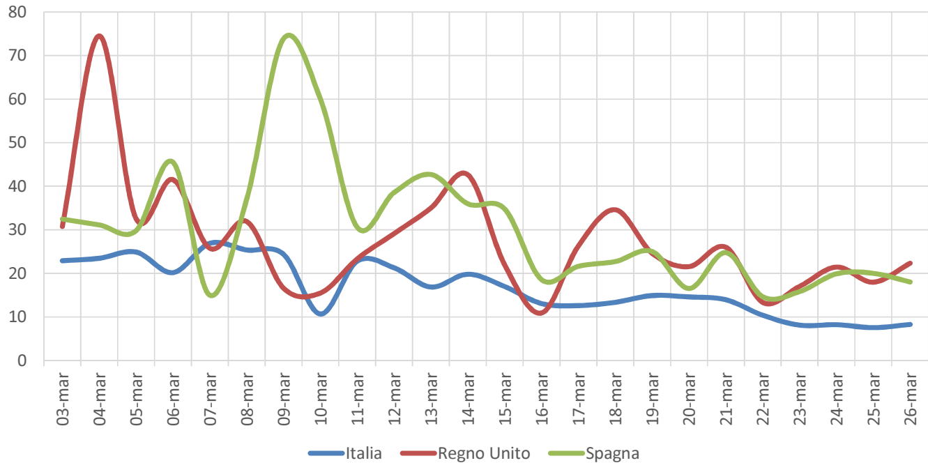
Fig. 10 - Confronto tra tasso di crescita giornaliero (%) del numero di contagiati confermati in 3 Paesi (dati del 27 marzo 2020)
