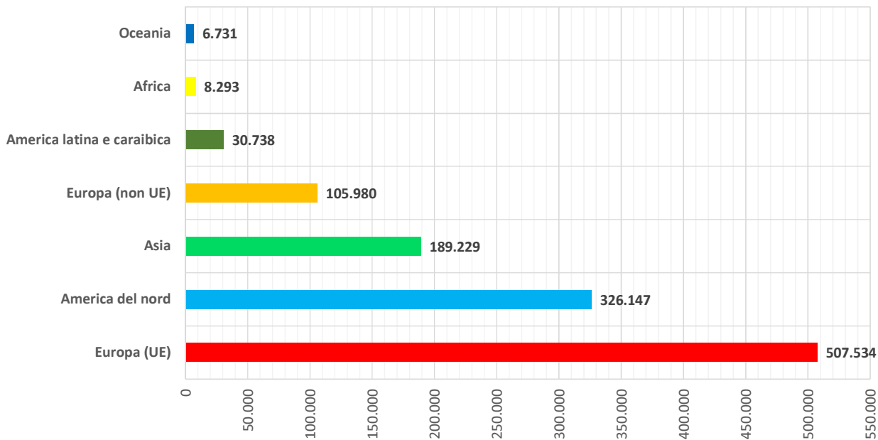
Fig. 5 - Numero del totale di contagiati confermati per continente (dati del 5 aprile 2020)
