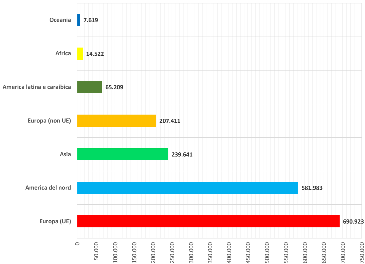
Fig. 5 - Numero del totale di contagiati confermati per continente (dati del 13 aprile 2020)
