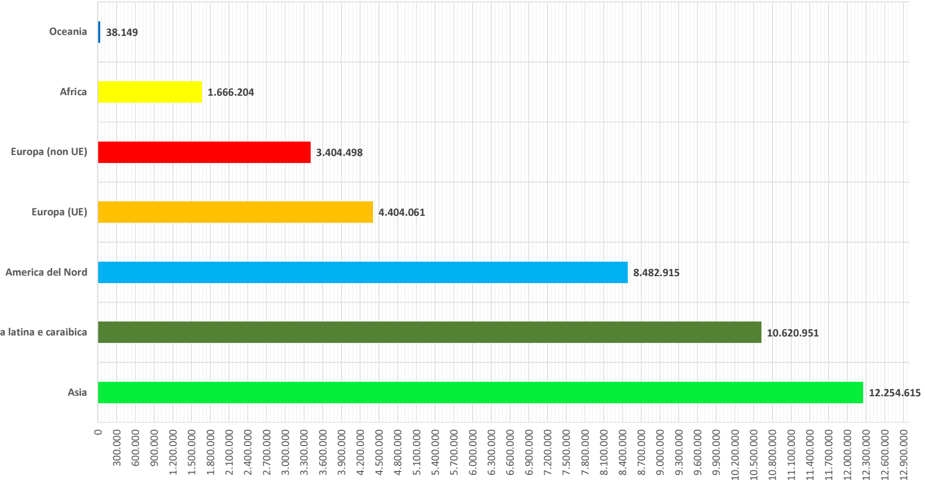
Fig. 4 - Numero del totale di contagiati confermati per continente (dati del 21 ottobre 2020)
